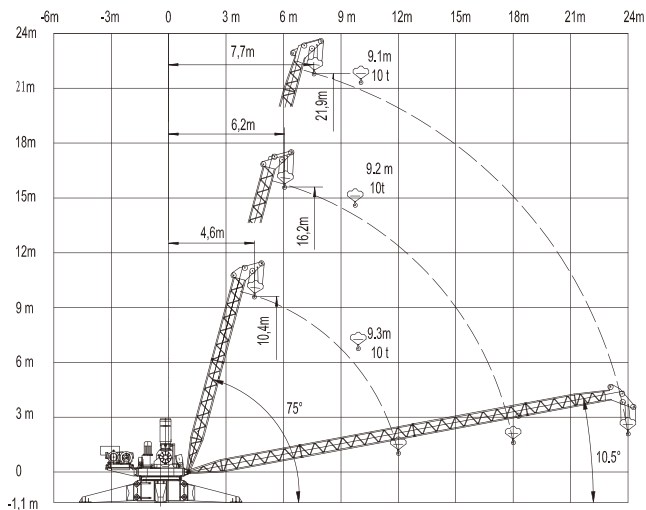
Подъемная стрела
